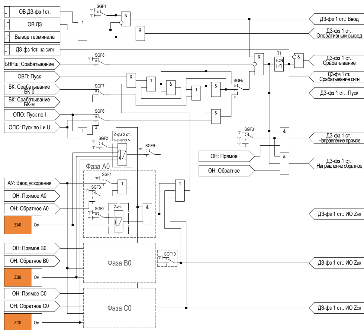
Рисунок 1.12 – Функциональная схема «ДЗ-фз 1ст.»
